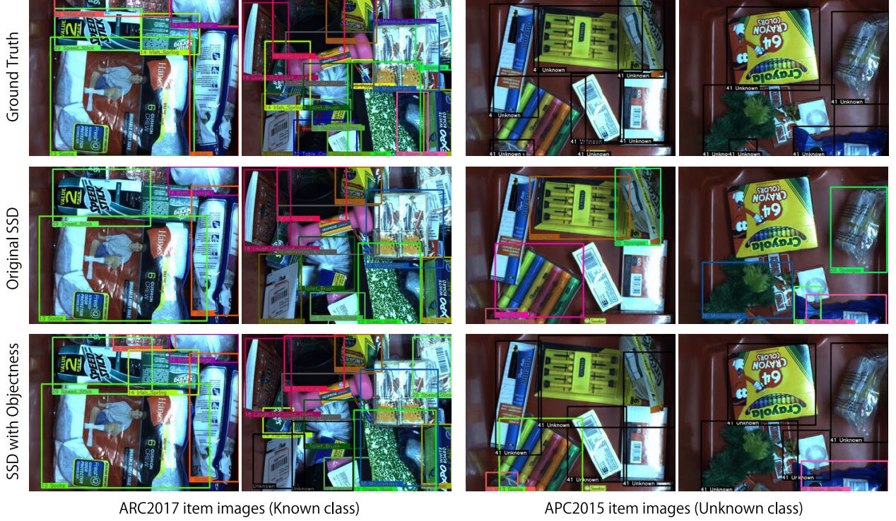
図 4 SSD と提案手法による検出結果例.
