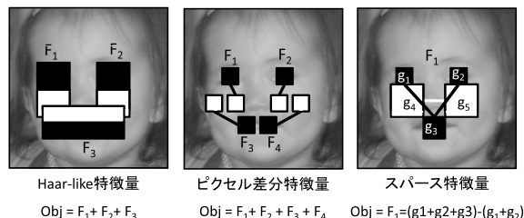
図 13: 特徴量の表現力の比較
