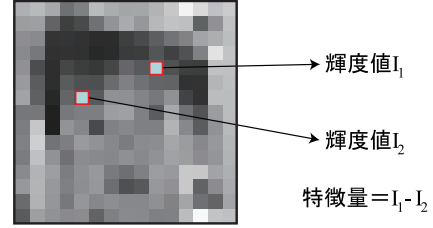
図 3: ピクセル差分特徴量
