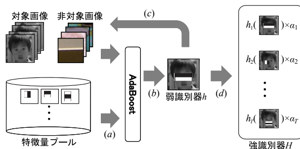
図 8: ブースティングによる学習の流れ
