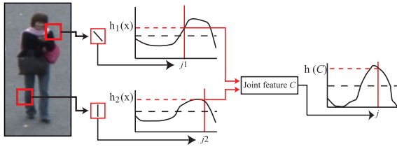
図 18: 共起確率特徴量
