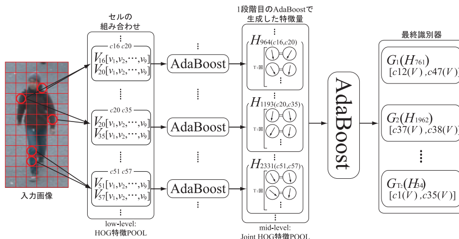
図 16: Joint HOG 特徴量
