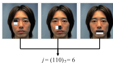
図 10: Joint Haar-like 特徴量
