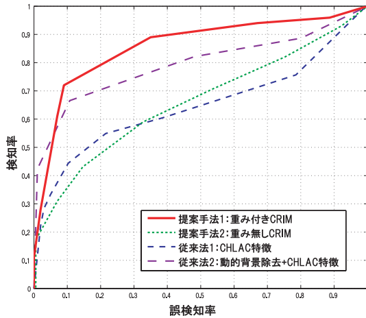
図 11: ROC カーブによる定量的評価
