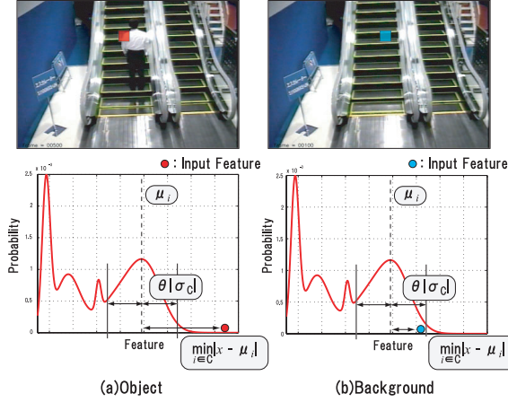
図 2: 混合正規分布モデルとの比較方法
