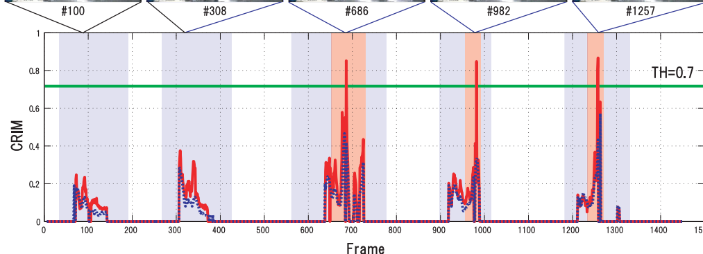
図 7: CRIM による異常行動検知結果
