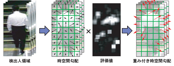
図 6: 重み付き時空間勾配を用いた CRIM 算出
