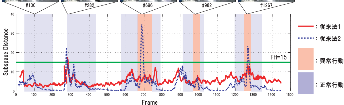
図 8: CHLAC による異常行動検知結果
